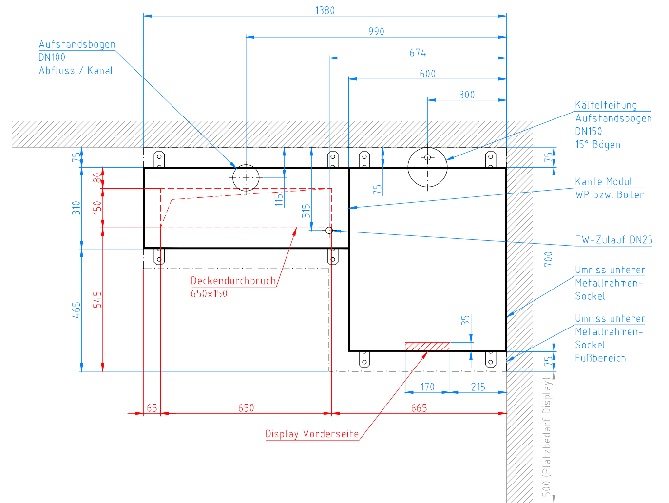
Fundamentplan SA-Etech Wärmepumpe + Hydrotower - Basis 6kW 200 oder 260 Liter Hydrotower 310mm tief auf linker Seite (90° gedreht)
