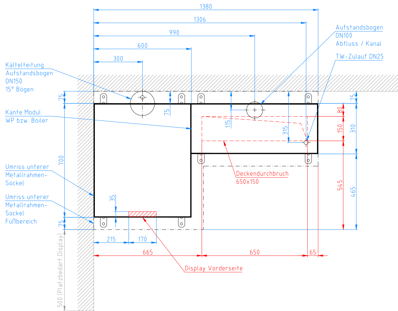
Fundamentplan SA-Etech Wärmepumpe + Hydrotower - Basis 6kW 200 oder 260 Liter Hydrotower 310mm tief auf rechter Seite (90° gedreht)
